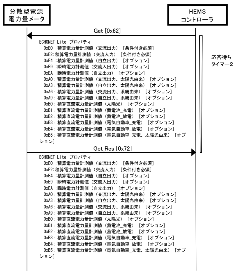
図 3-4 現在値取得のシーケンス例
