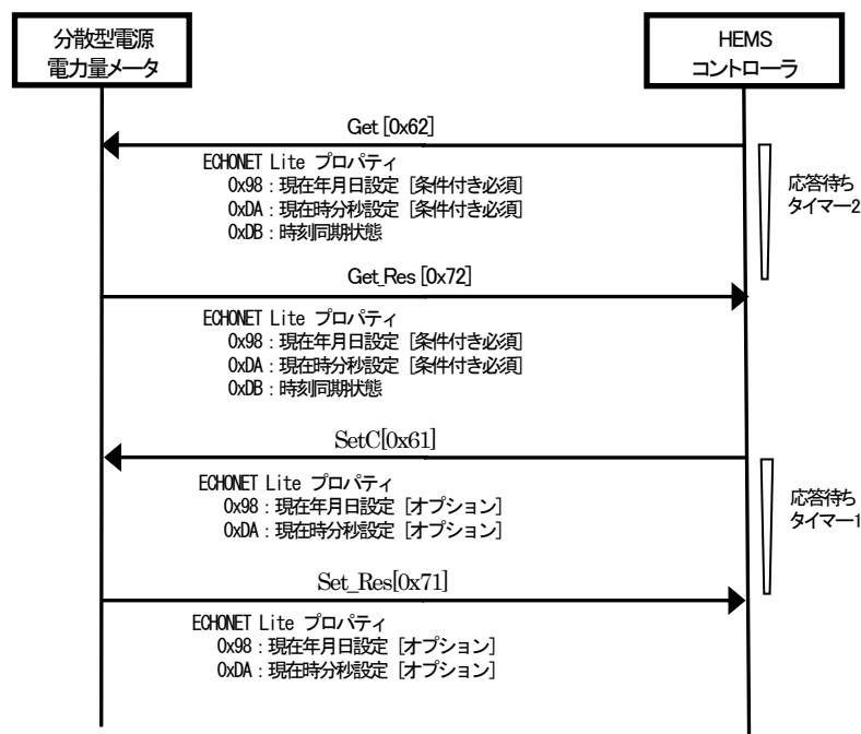
図 3-7 時刻同期例
