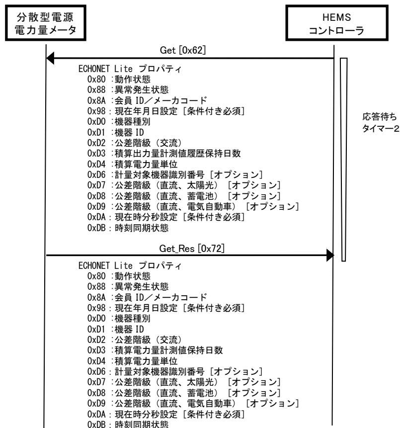
図 3-3 分散型電源電力量メータ属性情報等取得シーケンス例
