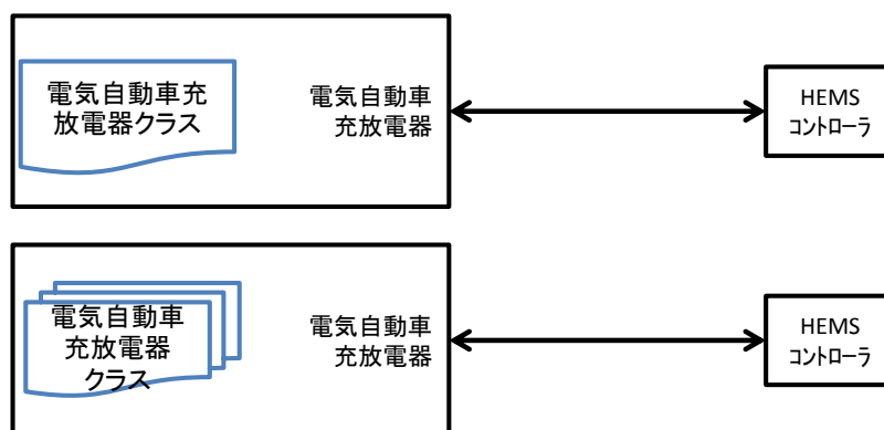
図 1-1 接続構成
