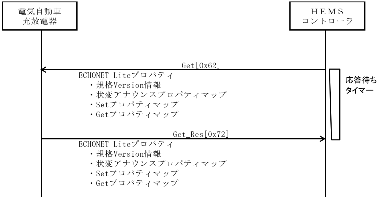
図 3-2 ECHONET Lite 属性情報取得シーケンス例
