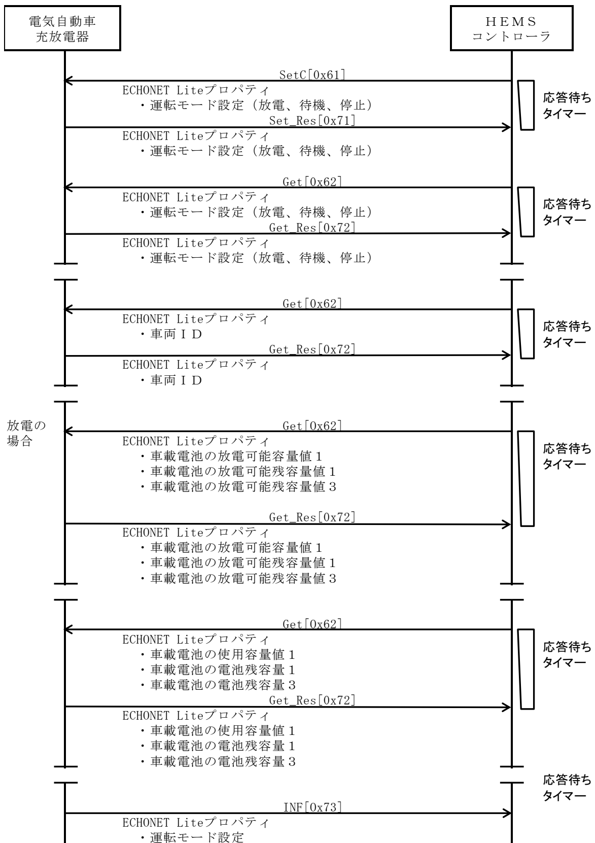
図 3-6 車両接続・充電不可・放電可時の操作シーケンス例
