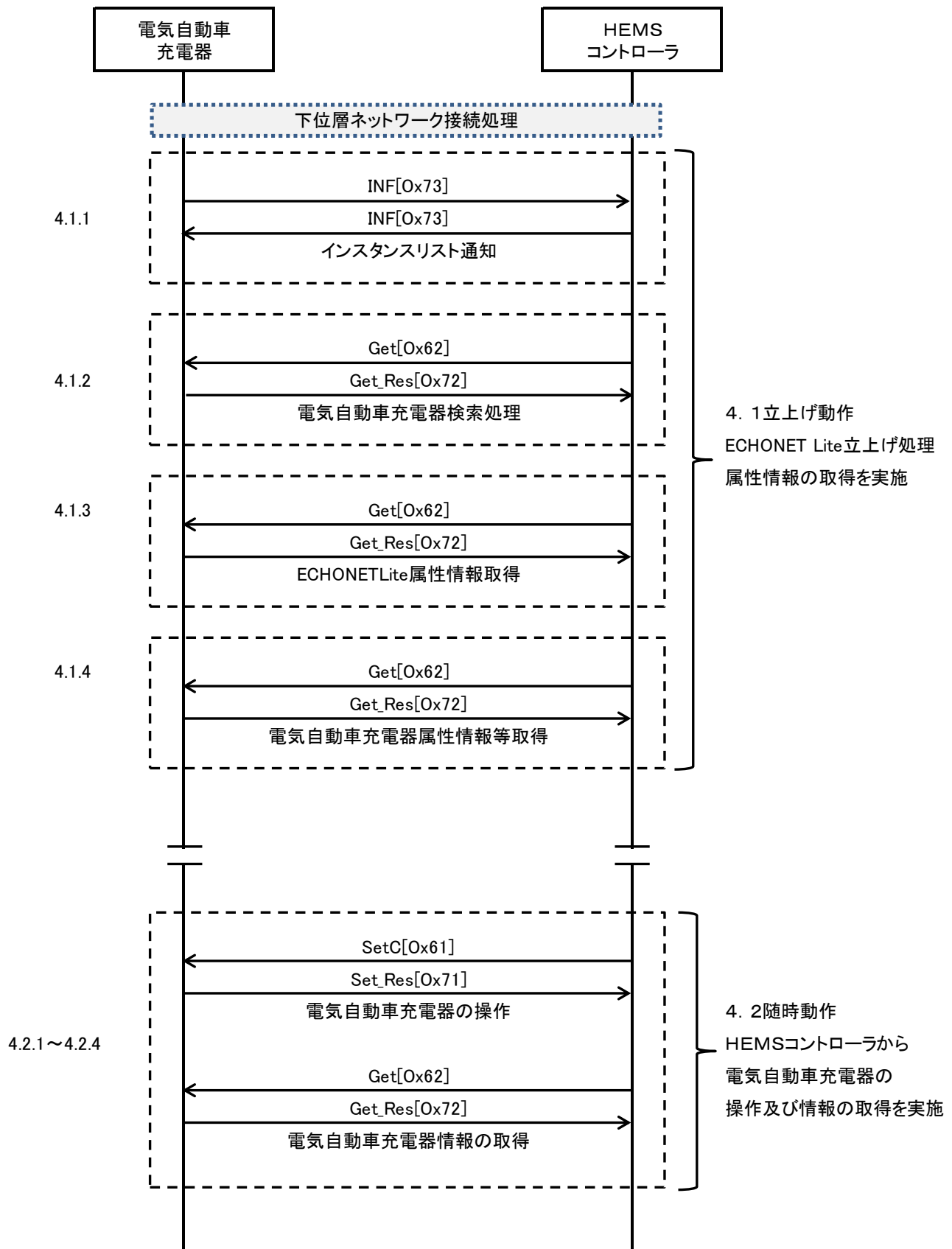
図 4-1 標準的な動作シーケンス例
