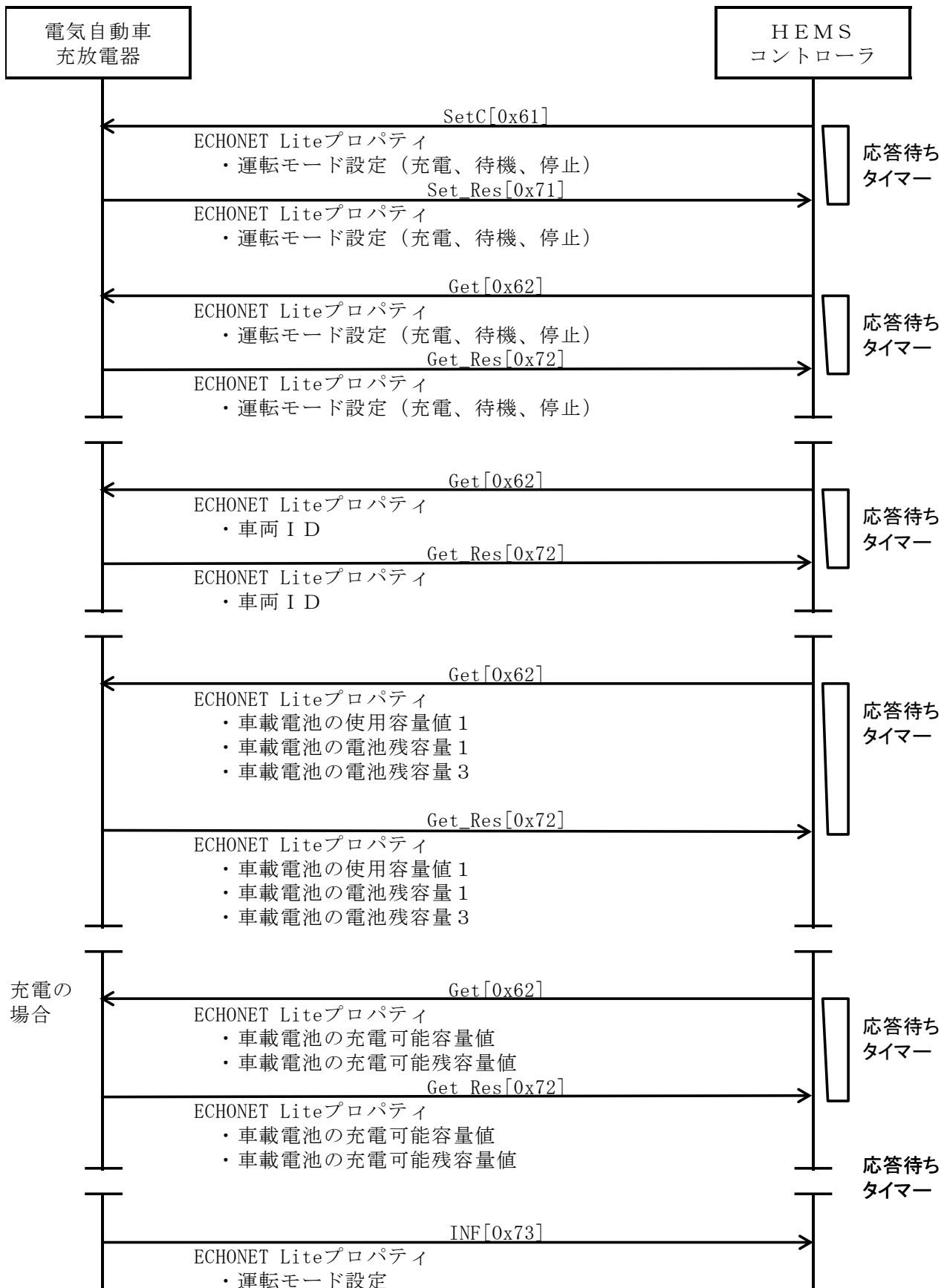
図 3-5 車両接続・充電可・放電不可時の操作シーケンス例
