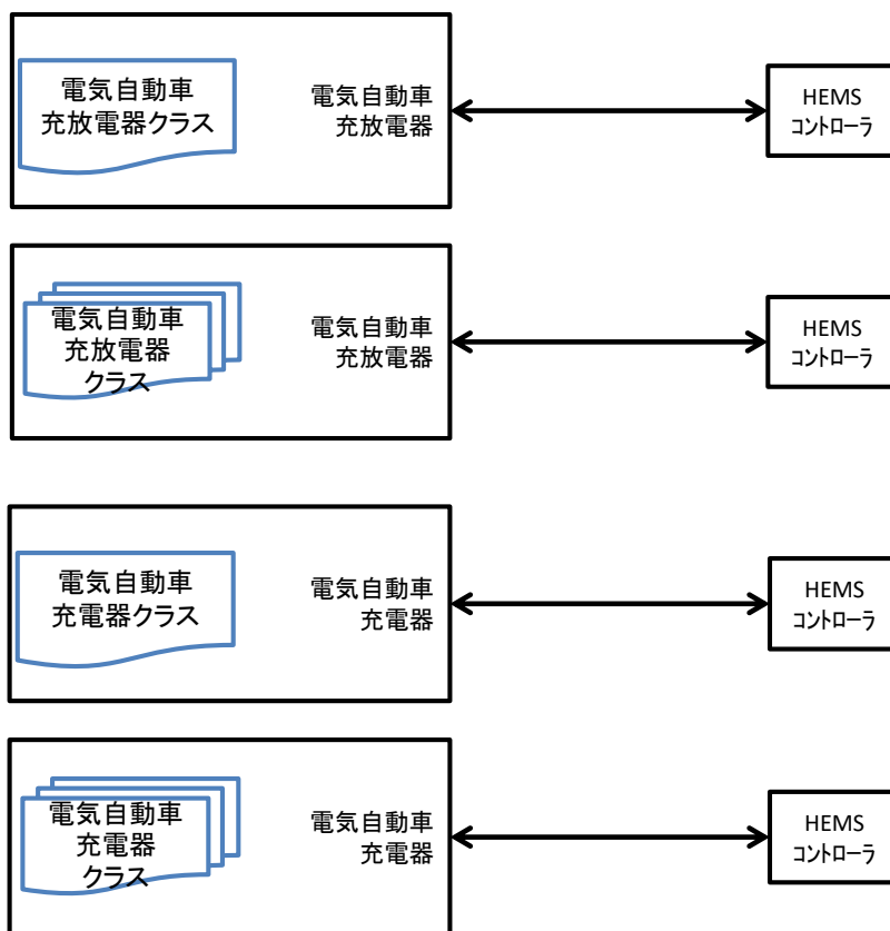
図 1-1 接続構成
