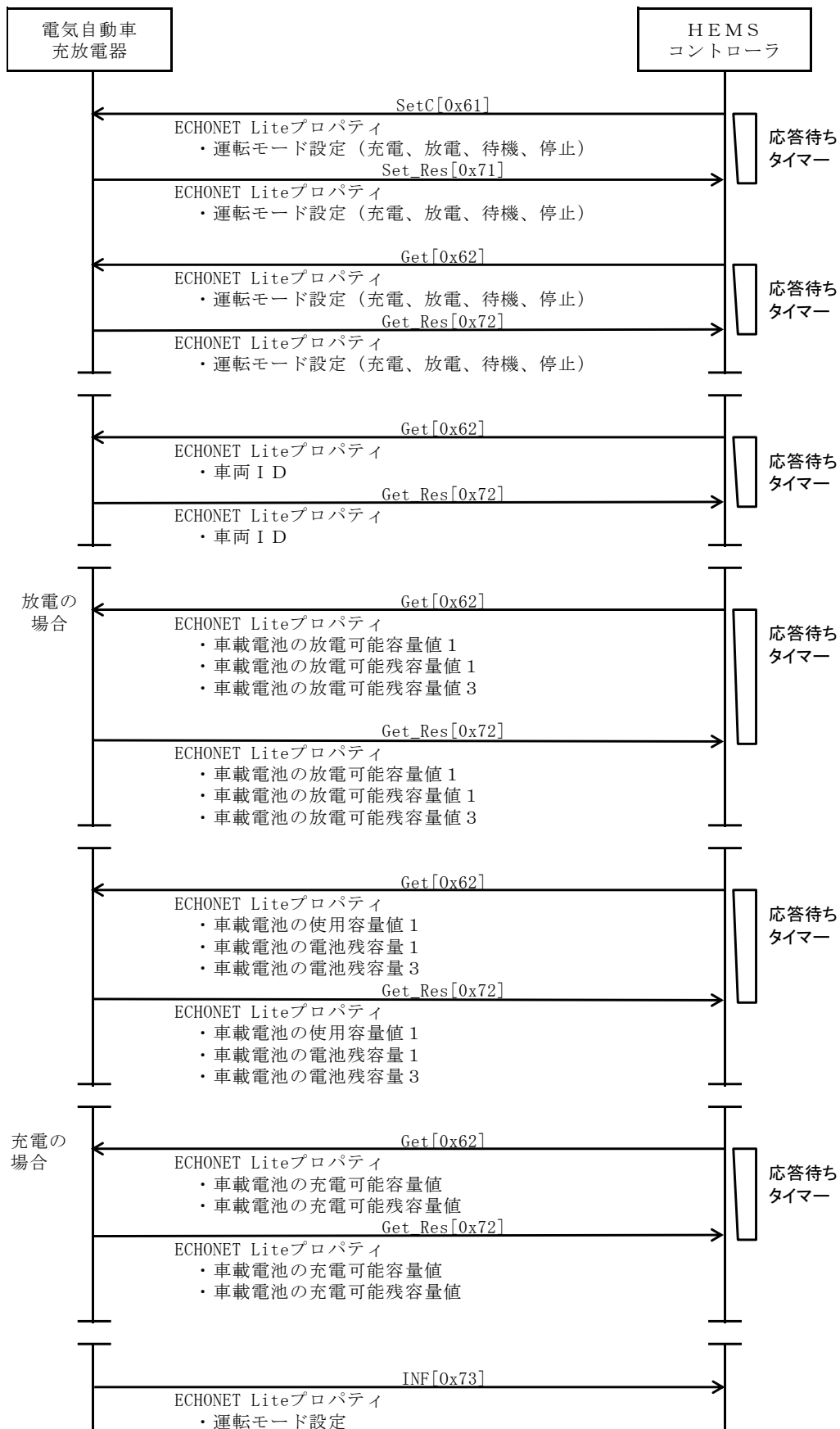
図 3-7 車両接続・充電可・放電可時の操作シーケンス例
