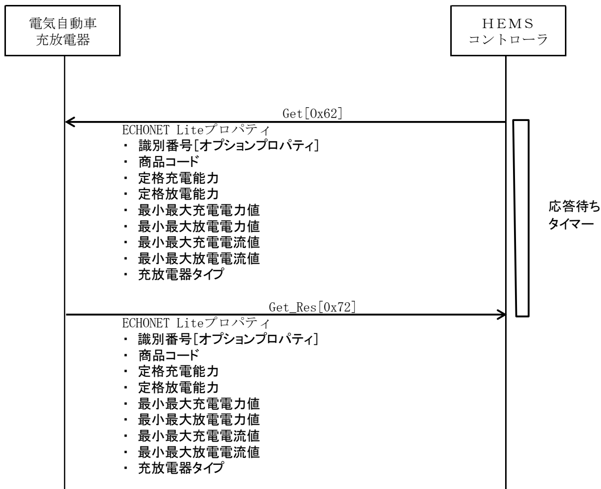
図 3-3 電気自動車充放電器属性情報等取得シーケンス例
