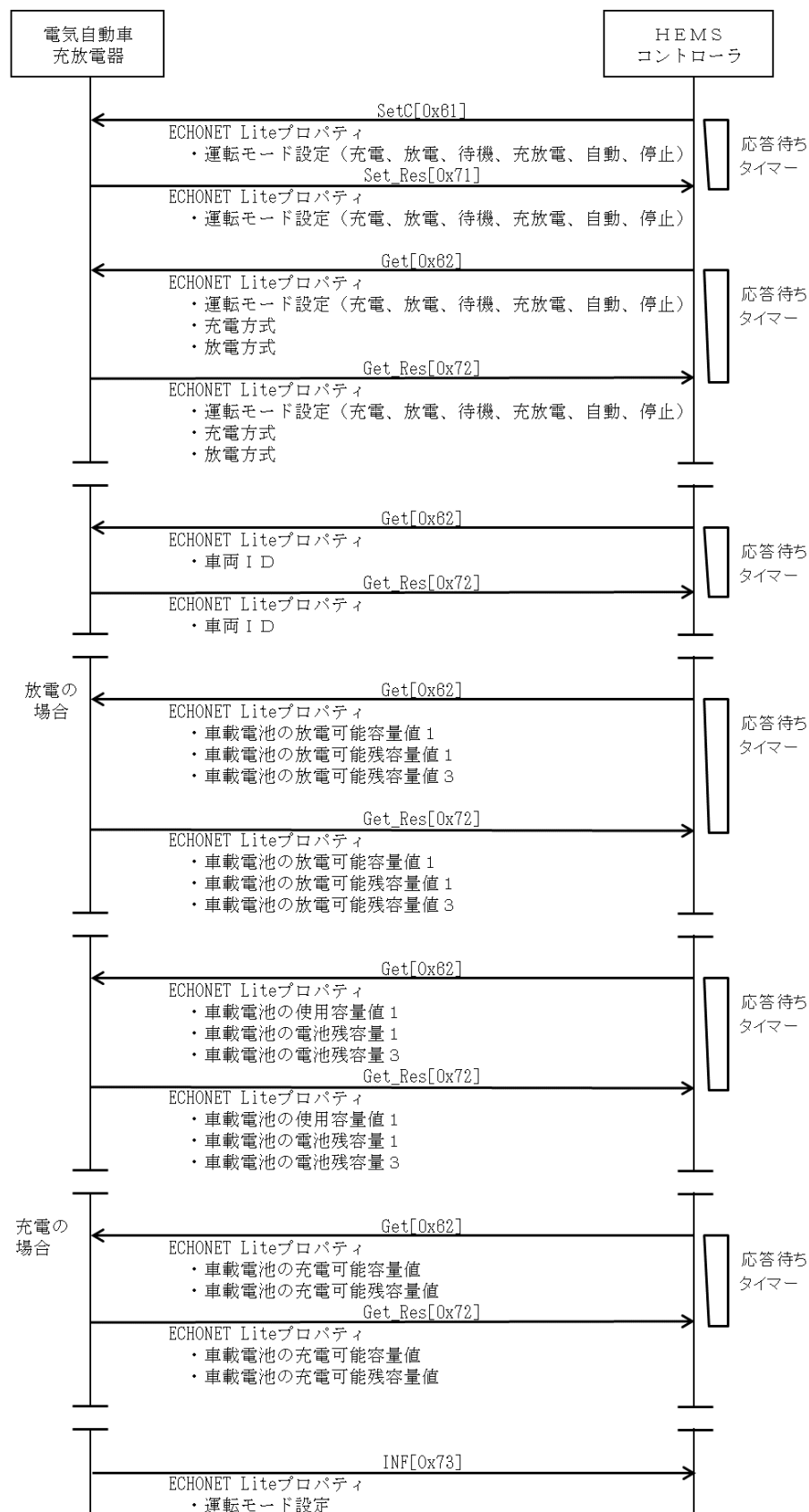
図 3-7 車両接続・充電可・放電可時の操作シーケンス例
