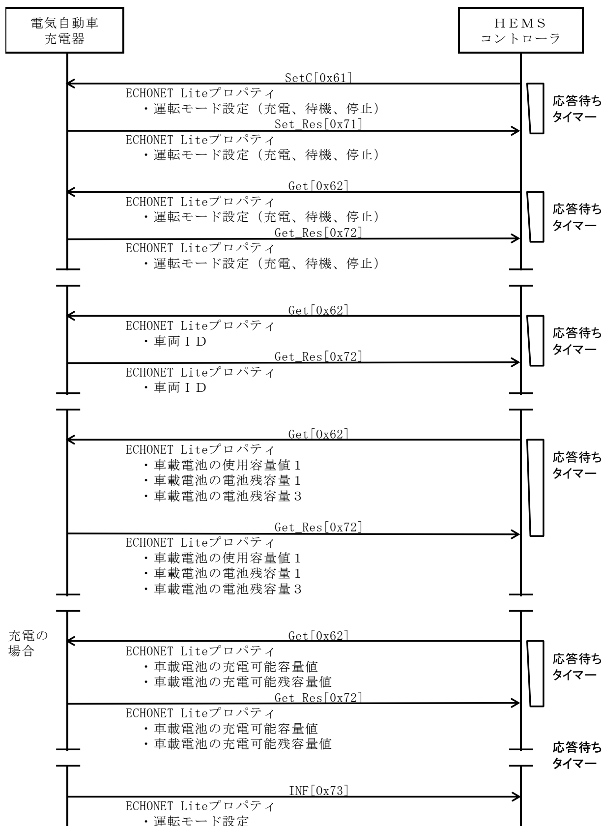
図 4-5 車両接続・充電可時の操作シーケンス例
