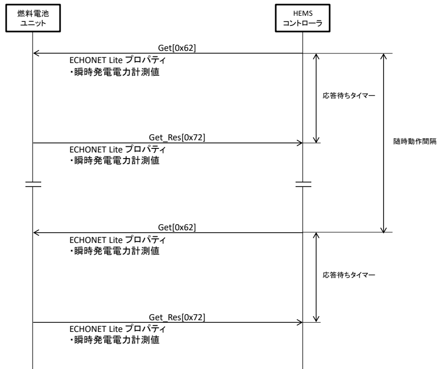
図 3-4 瞬時発電電力計測値取得シーケンス例
