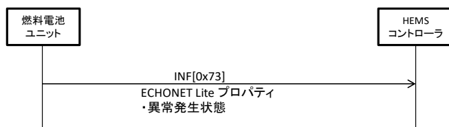
図 3-6 異常発生状態通知シーケンス例
