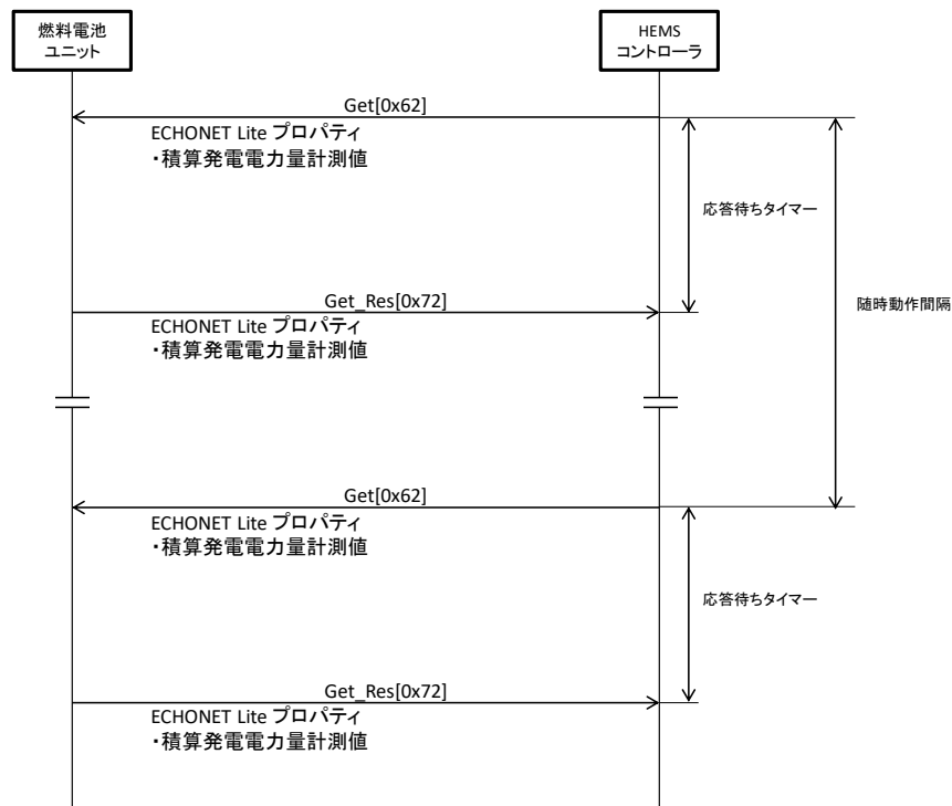
図 3-5 積算発電電力量計測値取得シーケンス例
