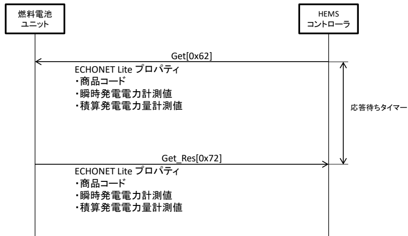
図 3-3 燃料電池属性情報等取得シーケンス例
