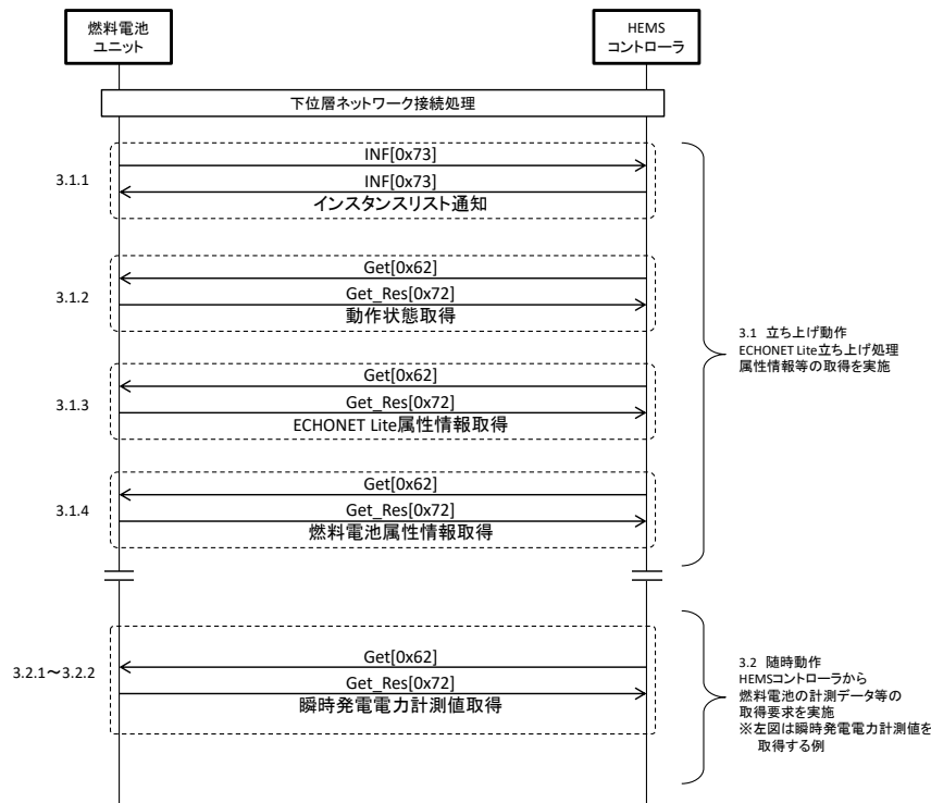
図 3-1 標準的な動作シーケンス例
