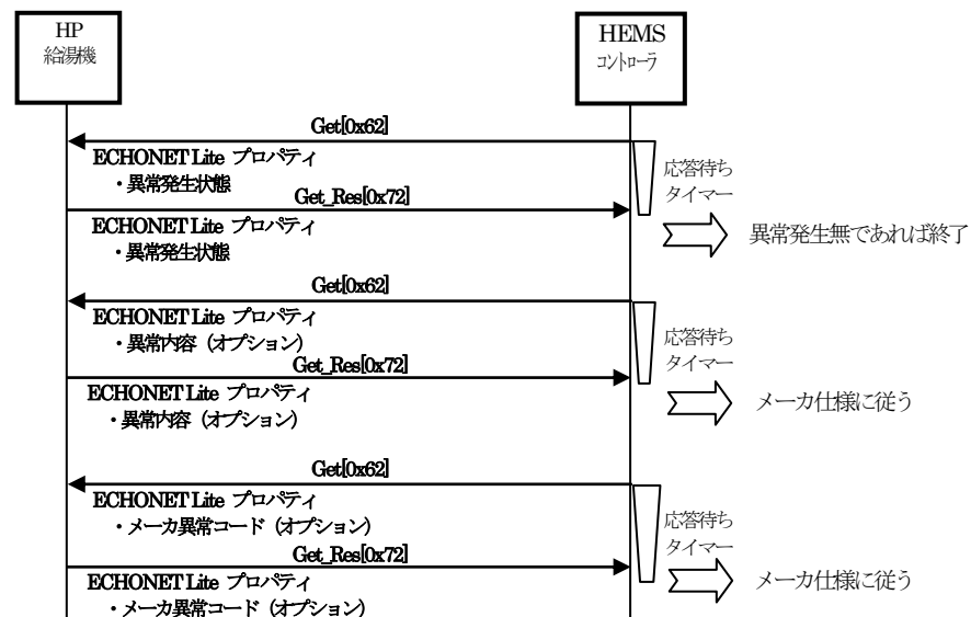
図 5-2 異常状態詳細情報取得
