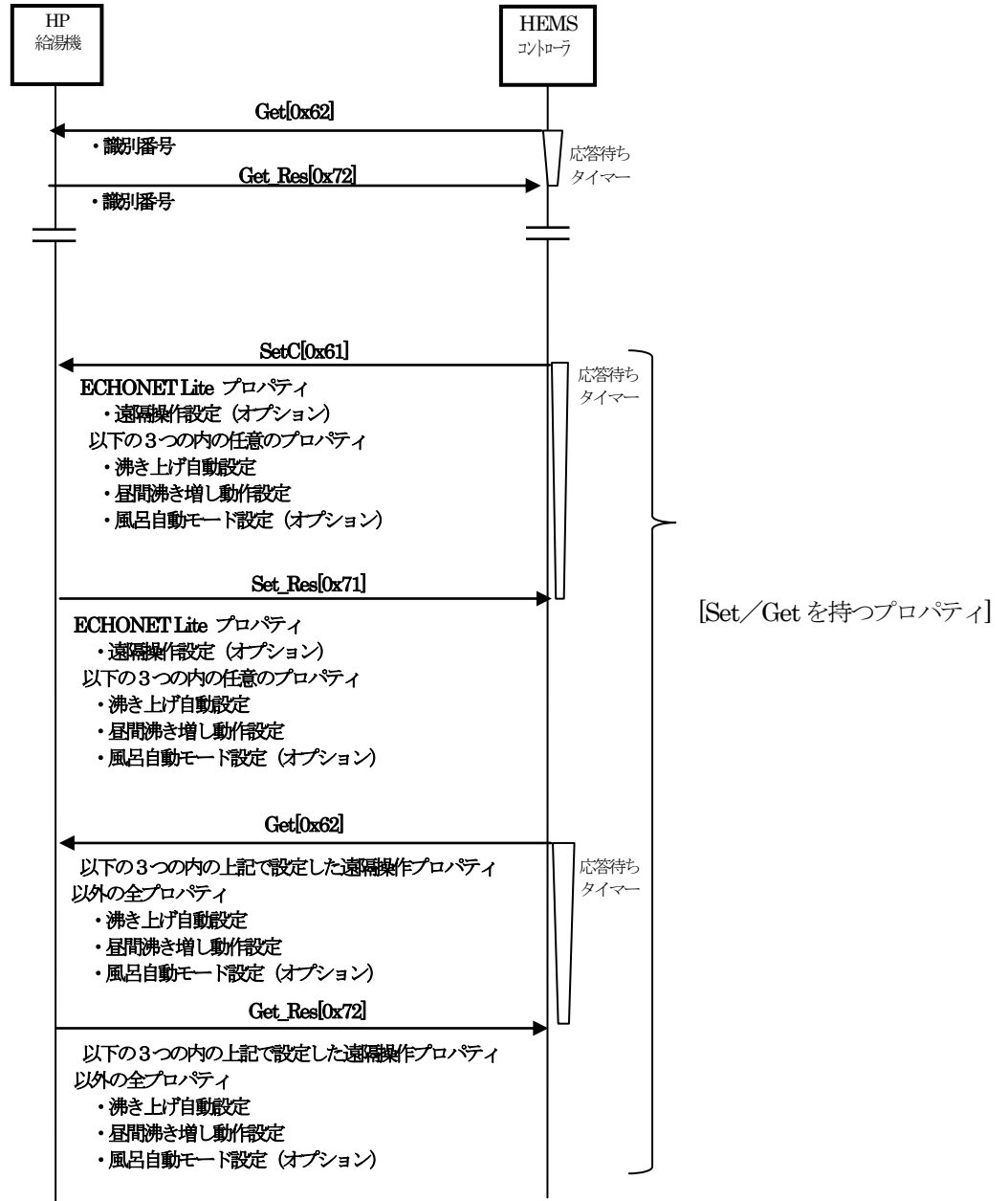
図 4-2 遠隔操作シーケンス(複数 OPC 設定)
