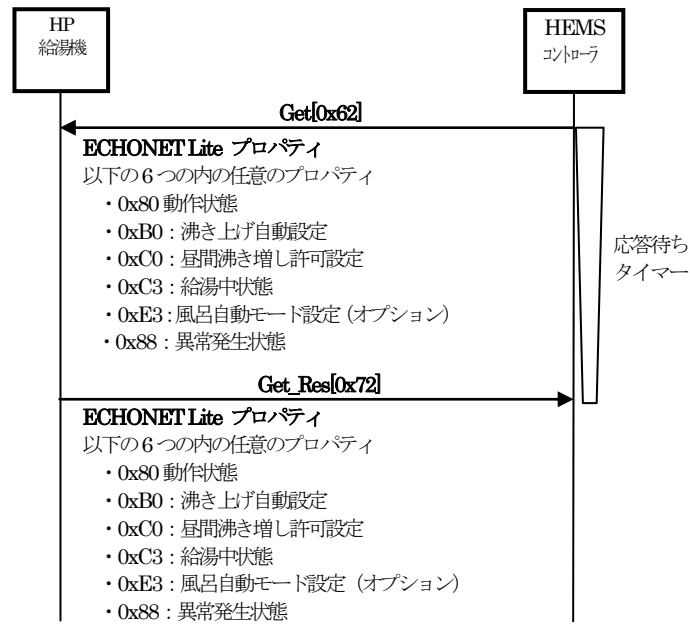
図 3-3 HP 給湯機状態取得シーケンス
