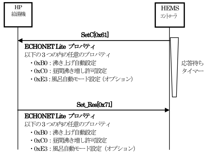
図 3-4 HP 給湯機設定、制御シーケンス
