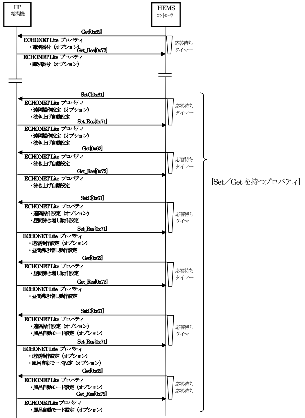
図 4-1 遠隔操作シーケンス(単独設定)
