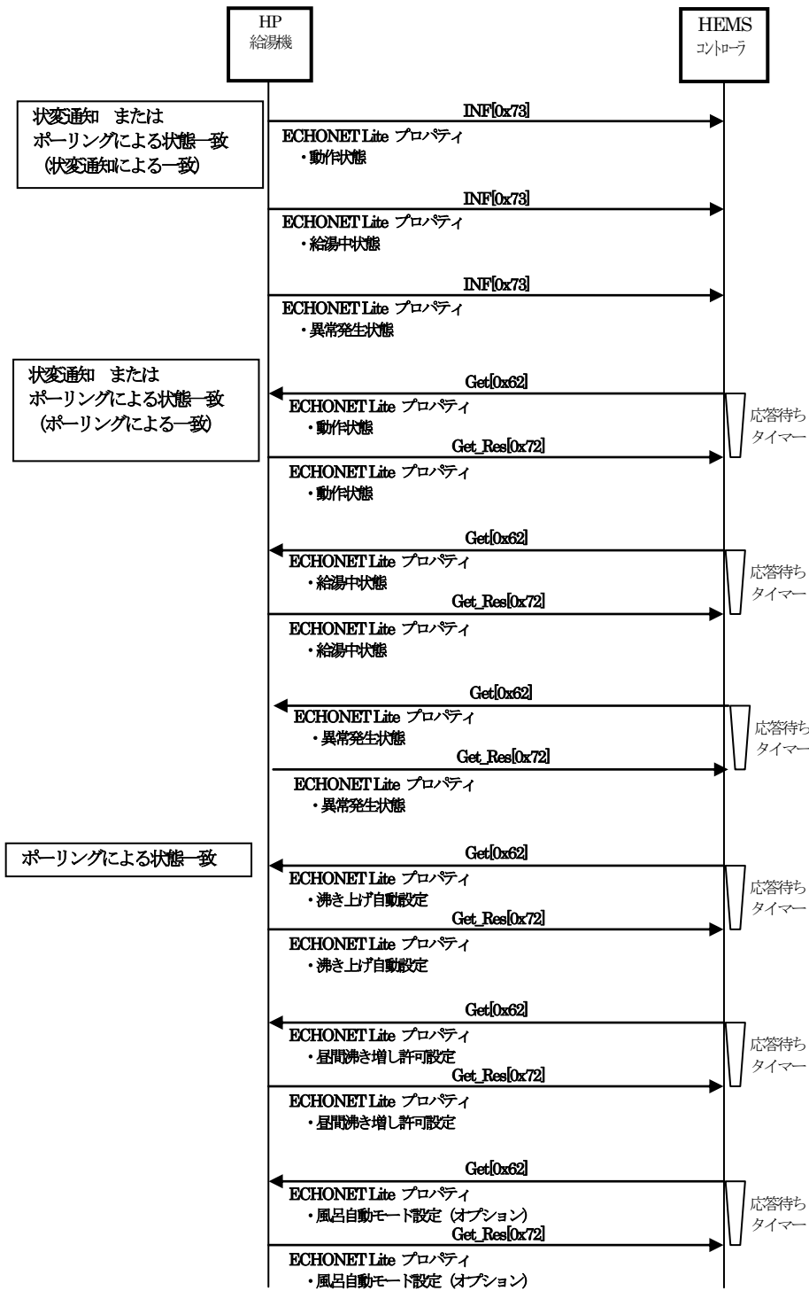
図 5-1 HEMS コントローラによる状態一致フロー
