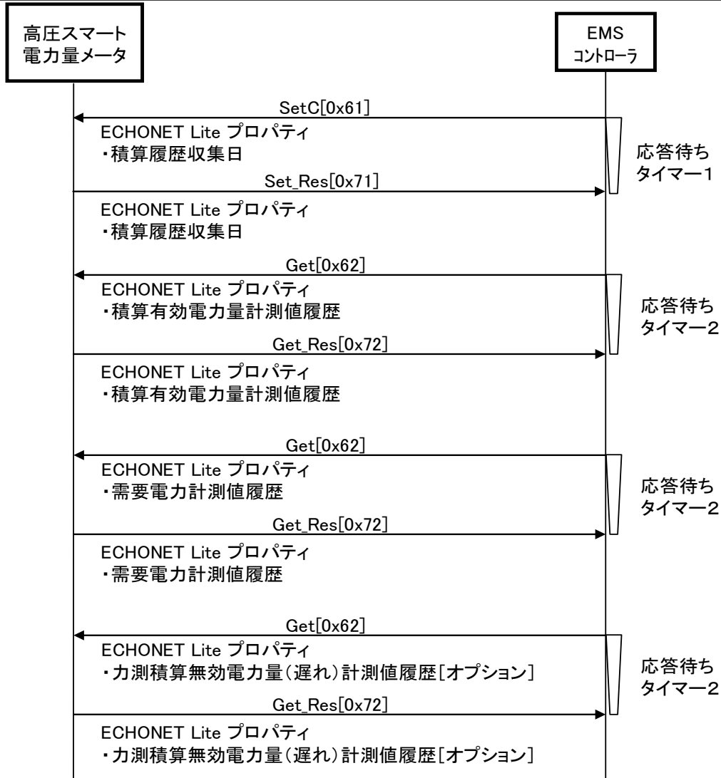
図 3-7 計測値履歴取得シーケンス例
