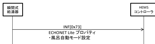
図 3-9 風呂自動モード設定状態変更通知シーケンス例
