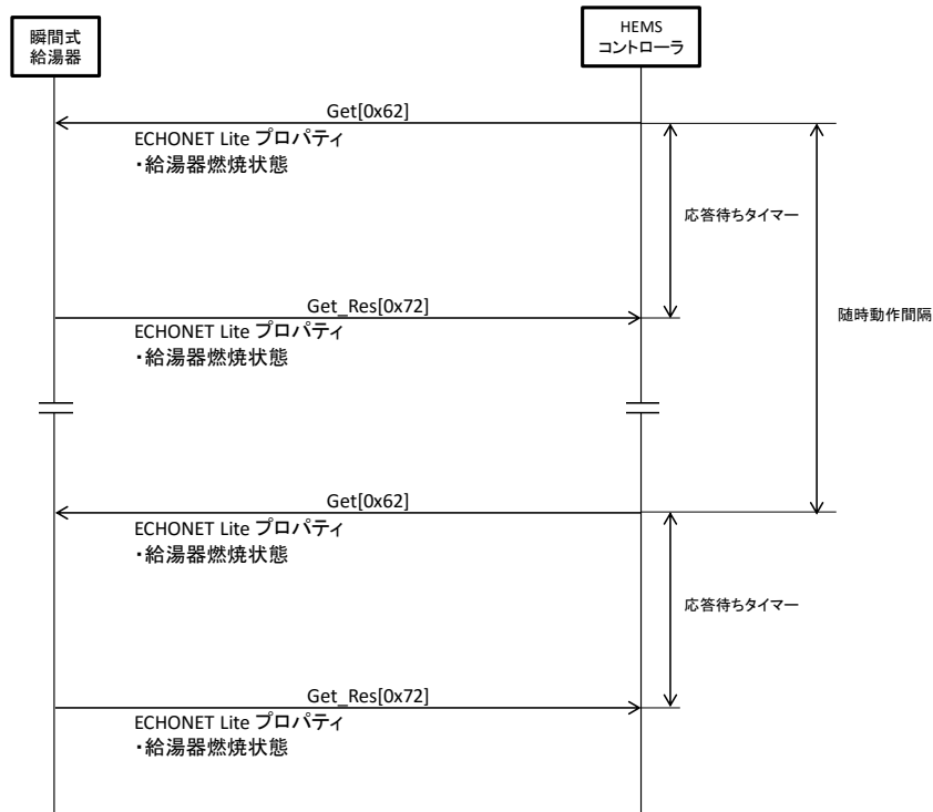
図 3-5 給湯器燃焼状態取得シーケンス例
