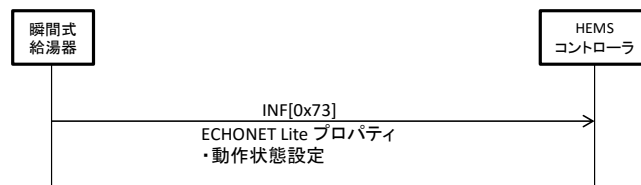
図 3-8 動作状態変更通知シーケンス例
