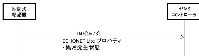
図 3-10 異常発生状態通知シーケンス例
