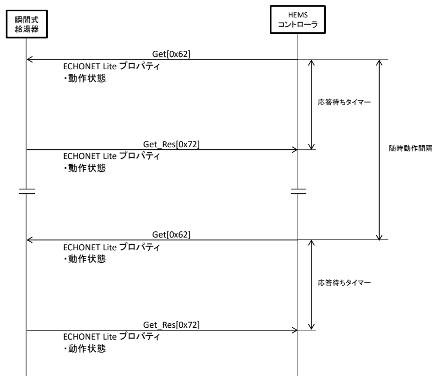
図 3-4 動作状態取得シーケンス例
