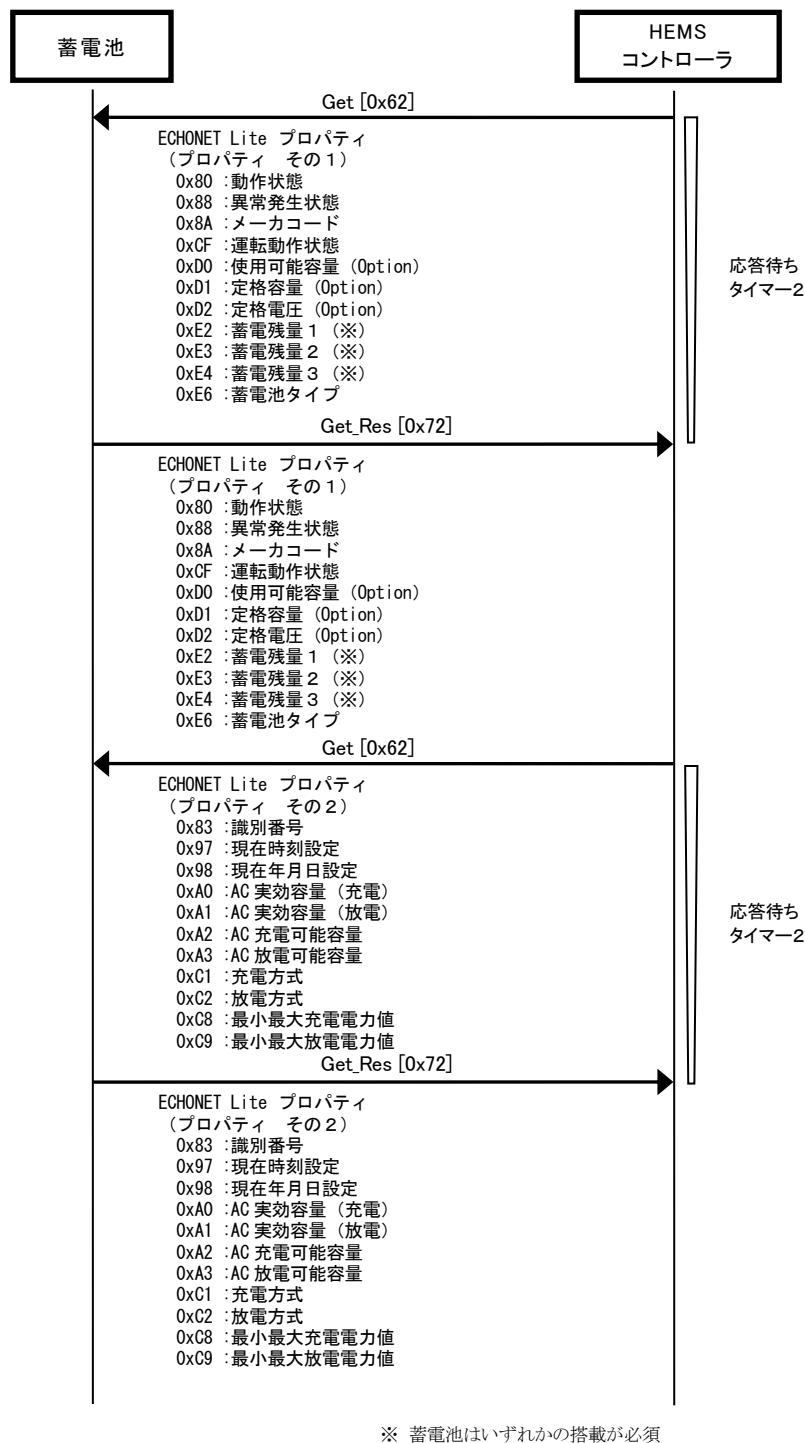
図 3-3 蓄電池属性情報等取得シーケンス例
