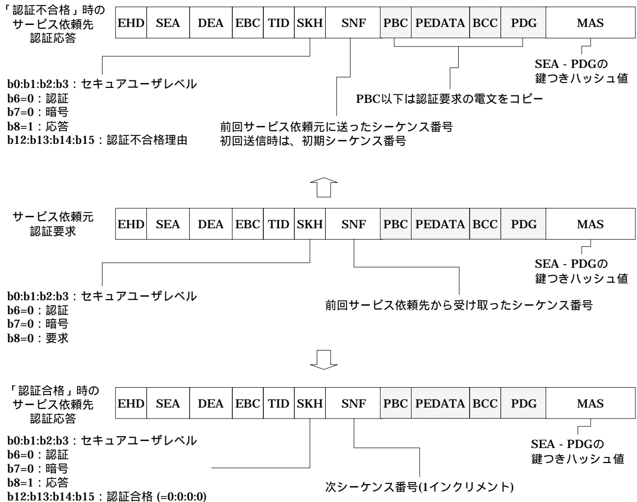
図10.14 ECHONET セキュアフレームと認証シーケンス (認証・暗号化電文形式)
