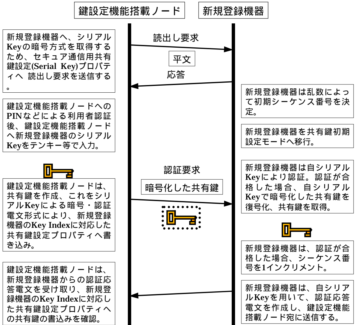
図10.19 セキュア通信用共有鍵 (User Key) 設定シーケンス
