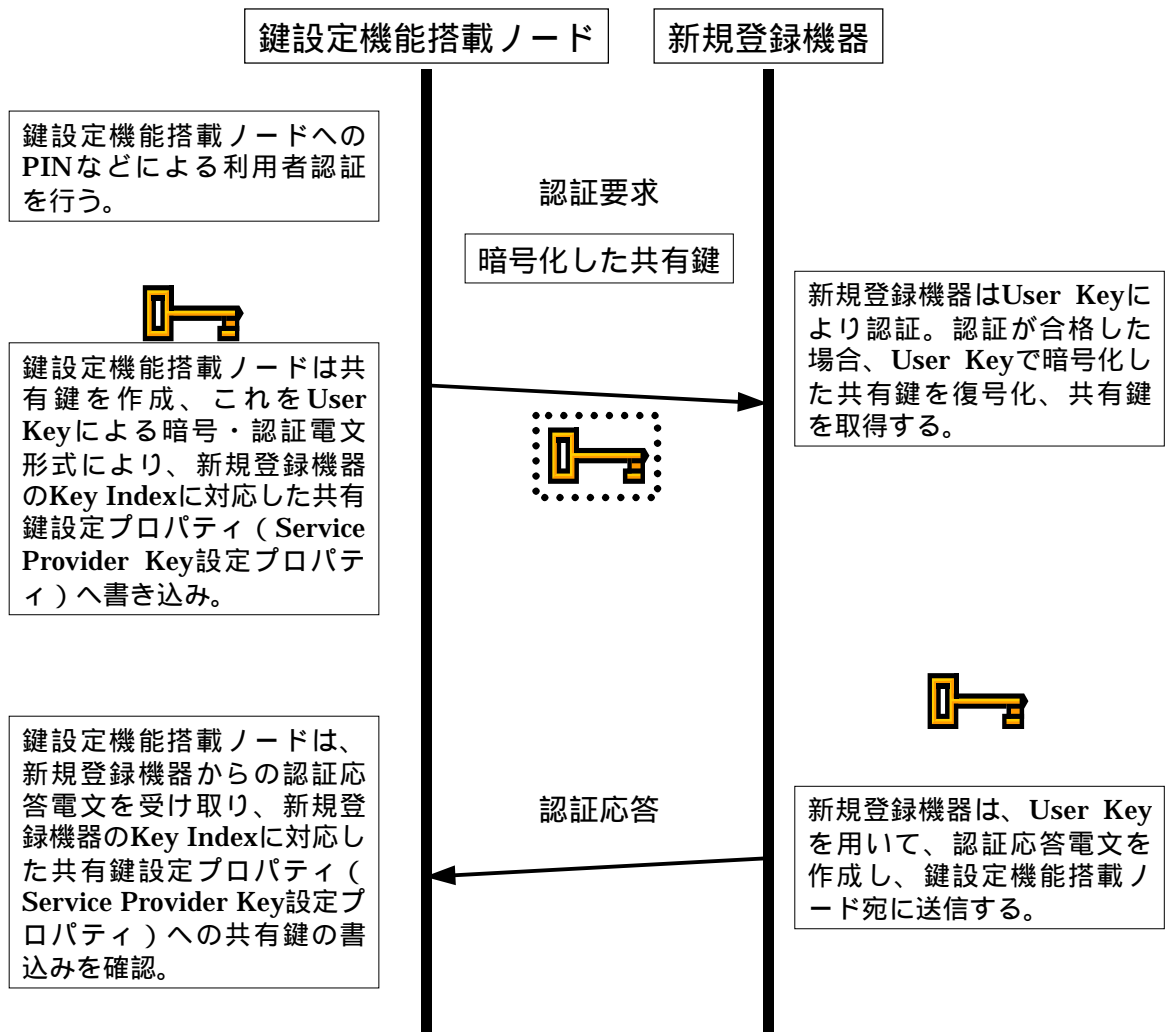
図10.21 セキュア通信用共有鍵 (Service Provider Key) 設定シーケンス
