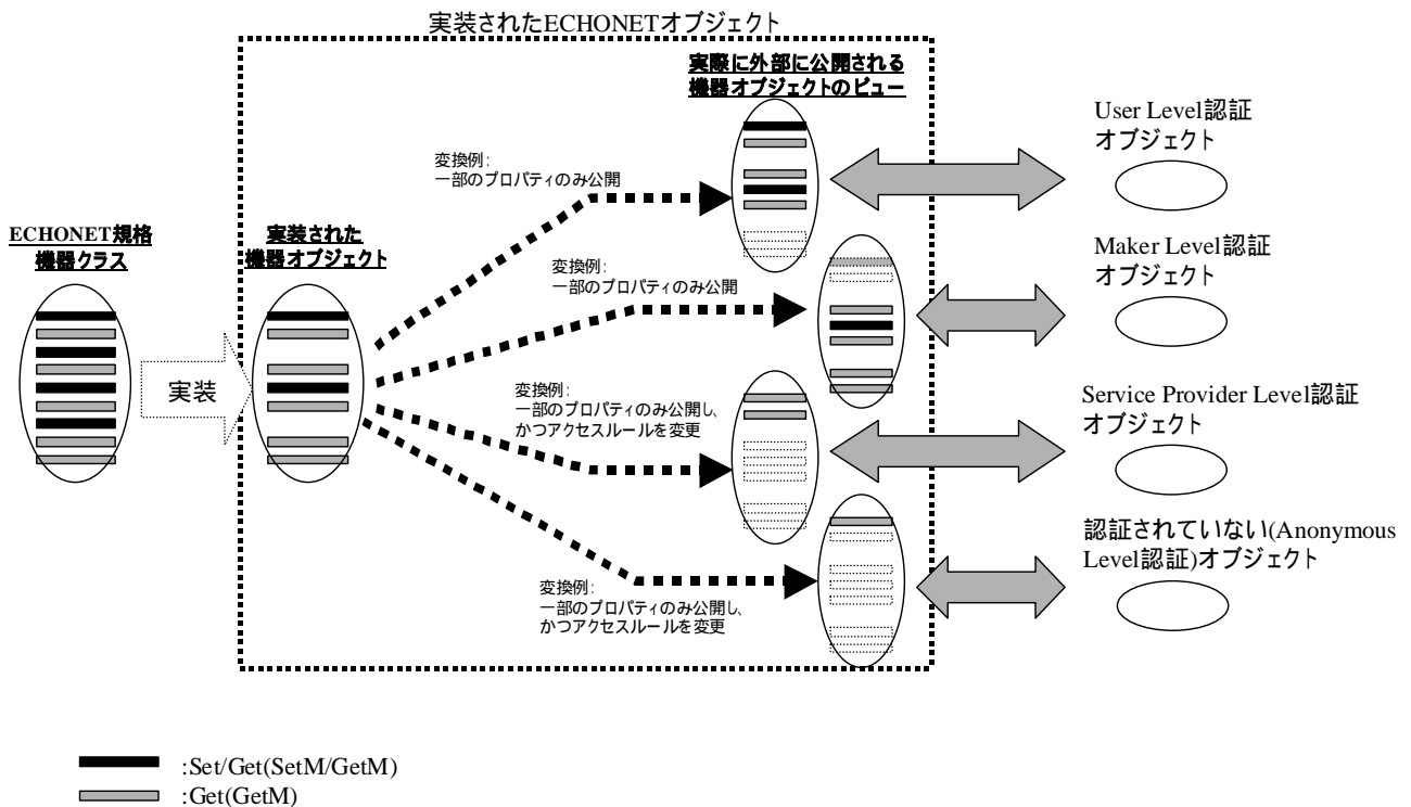
図10.27 機器オブジェクトを4つのアクセス制限レベルで実装した例
