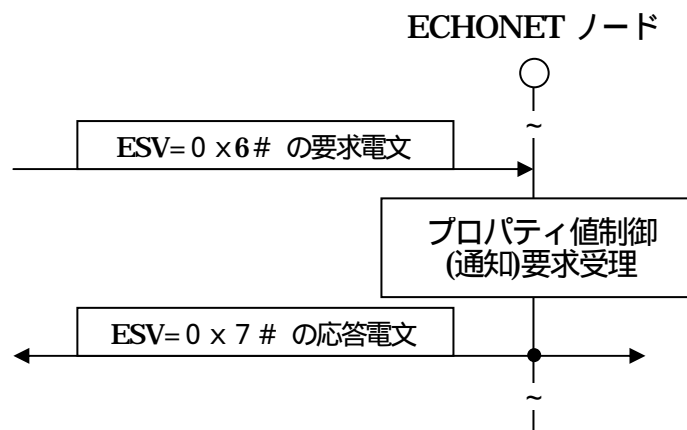
図5.5 ESV = 0x6 ( : 1 ~ 3, 5 ~ 7, 9, B, C, E) CpESV = 0x6 ( : 1, 2) 要求受信時の基本シーケンス
