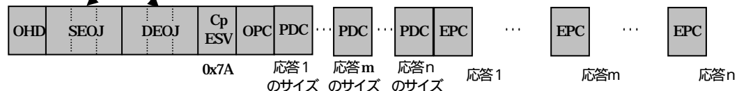
図 4 . 1 7 プロパティ値通知(応答要)とプロパティ値通知応答の関係
