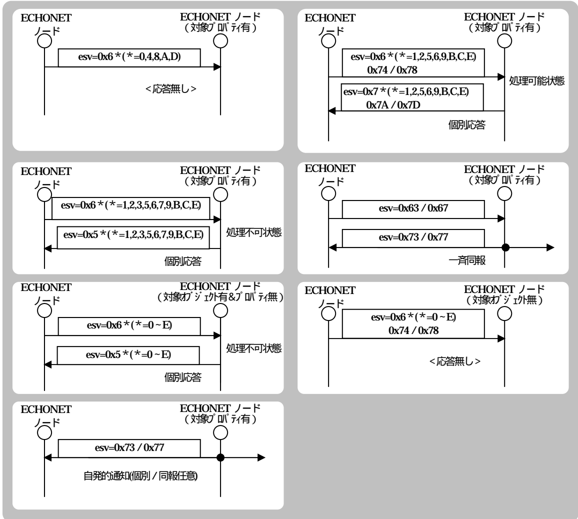
図 4 . 9 . 2 サービス関連基本シーケンス図
