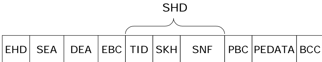
図10.7 暗号無し・認証無しの場合のフレームフォーマット
