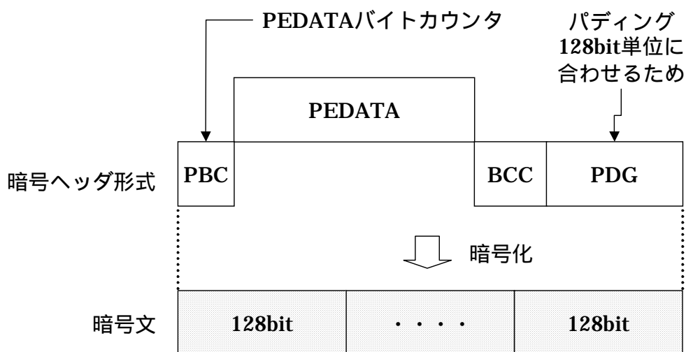
図10.13 セキュア電文形式における暗号化部分
