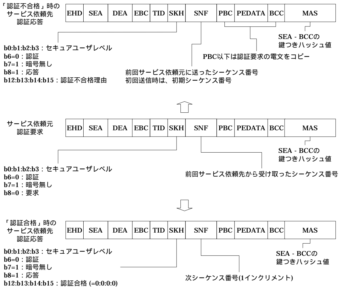
図 1 0 . 1 5 ECHONET セキュアフレームと認証シーケンス ( 認証・暗号化電文形式 )
