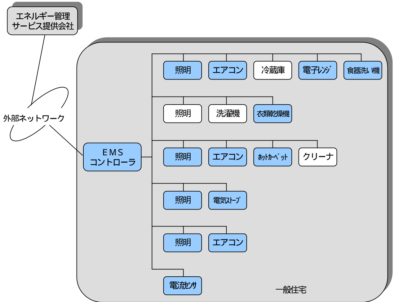
図7.1 住宅用EMSシステムとECHONET ネットワーク
