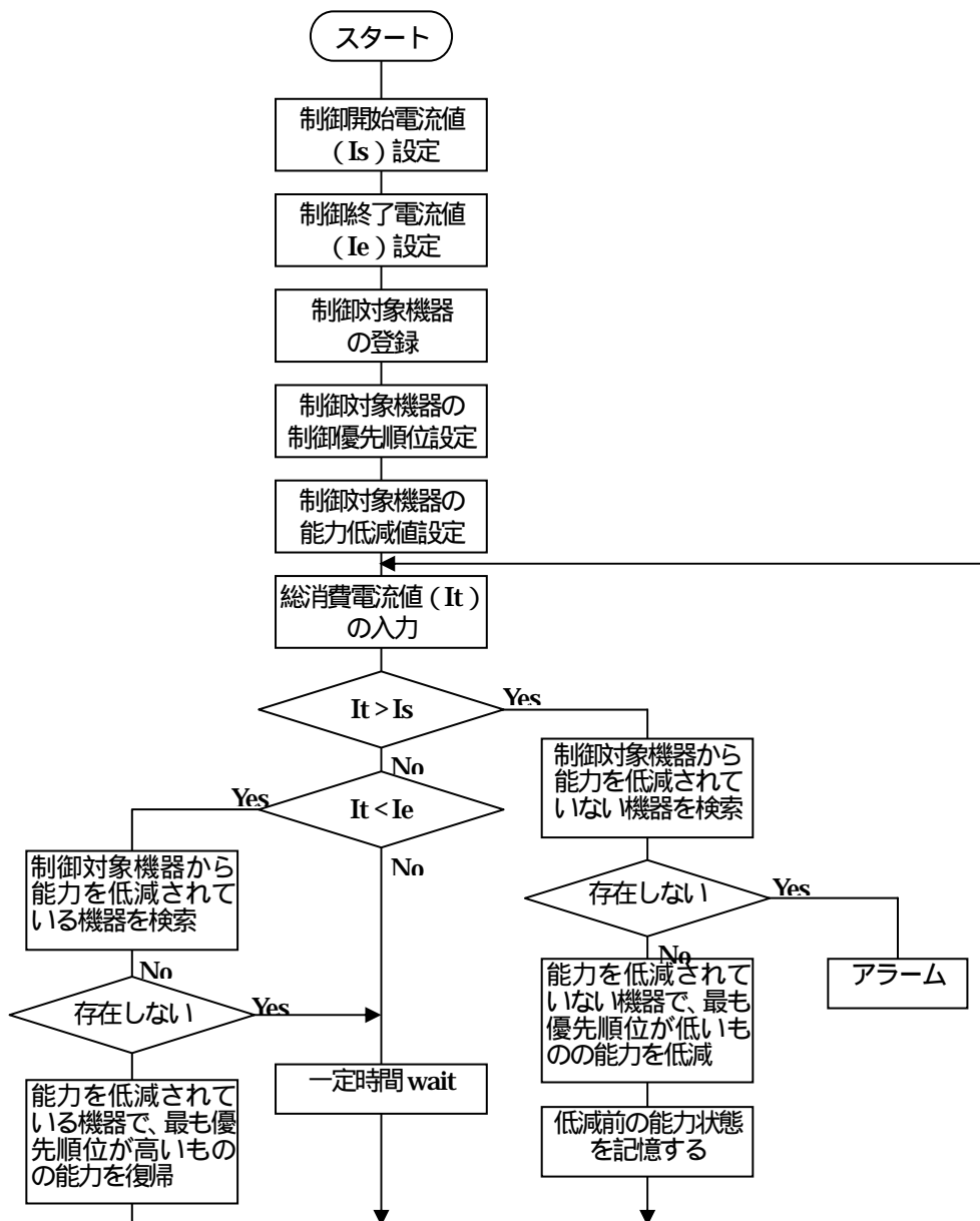
図 7.2 住宅用フィードバック方式ピークカット EMS の制御概要
