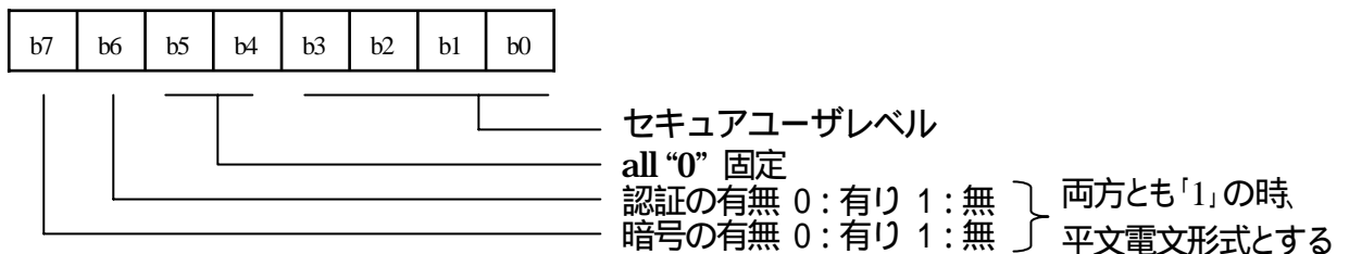
図 5 - 4 セキュア設定詳細
