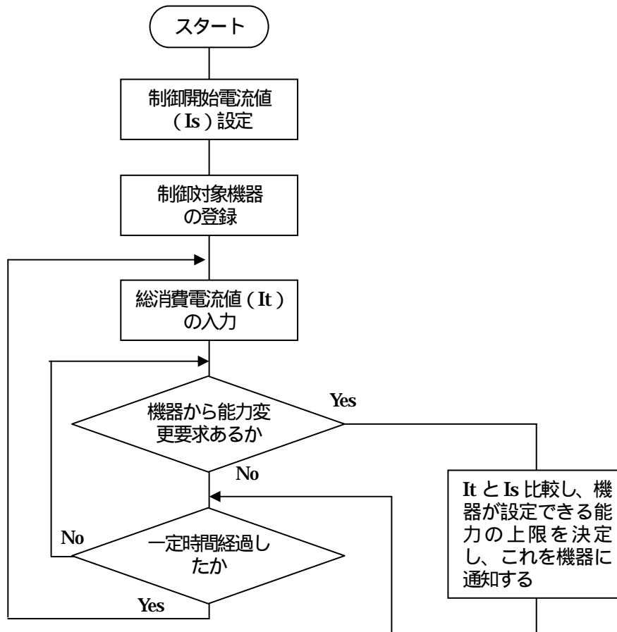
図7.3 住宅用フィードフォワード方式ピークカットEMSの制御概要
