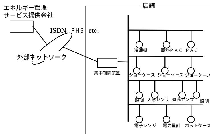
図 8 . 1 店舗 EMS の構成例
