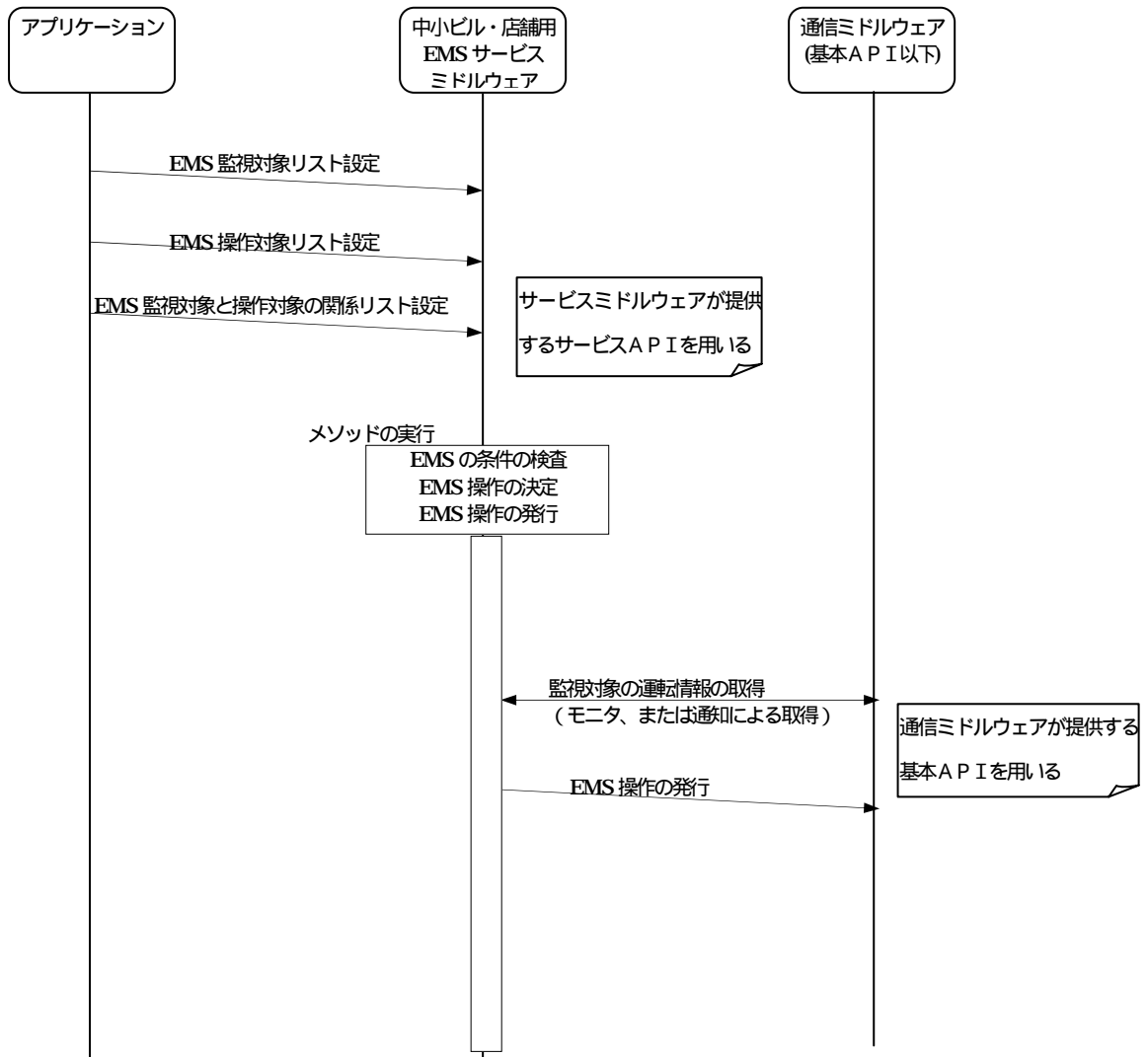
図 8.4 中小ビル・店舗用 EMS サービスミドルウェアの基本動作シーケンス
