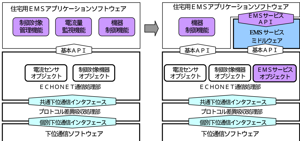
図7.5 住宅用EMS サービスミドルウェアとサービスオブジェクト
