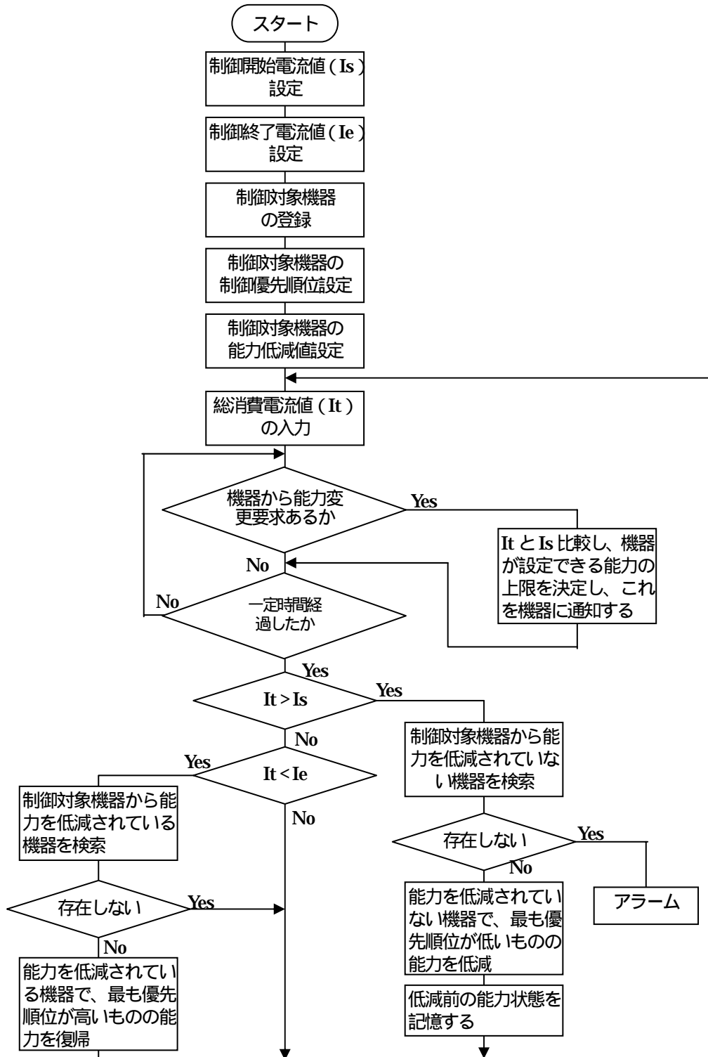
図7.4 住宅用フィードフォワード方式ピークカットEMSの制御概要
