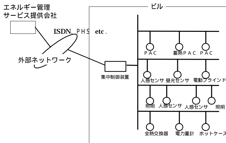
図 8 . 2 中小ビル EMS 構成例
