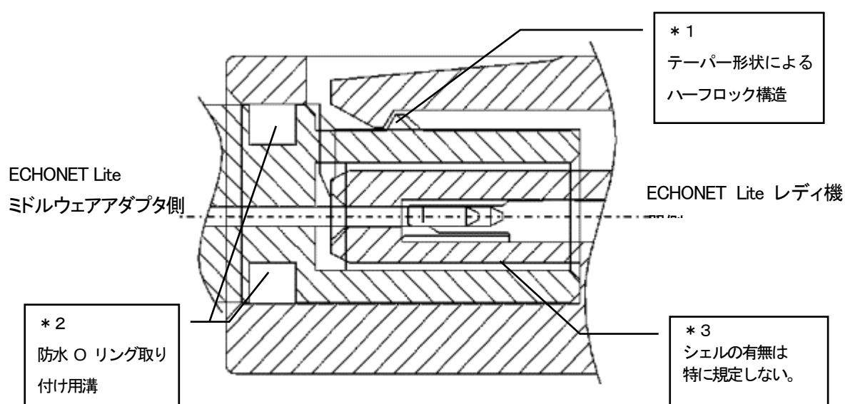
図3-7 (c) MA9 コネクタ 嵌合図
