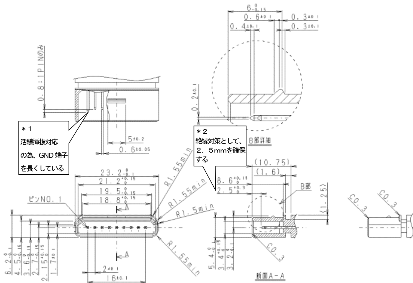
図3-7 (b) MA9 プラグ (ECHONET Lite ミドルウェアアダプタ側)
