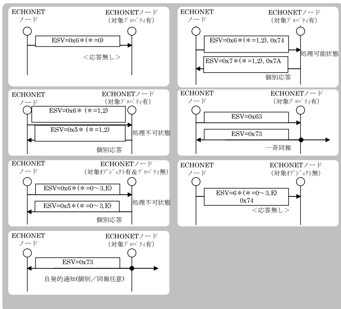
図 3-6 各 ESV 送受信時のシーケンス図
