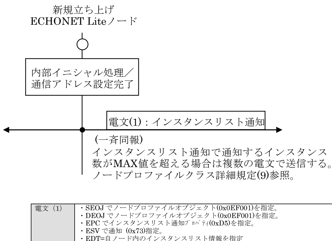
図 4-6 ECHONET Lite ノードスタート時の基本シーケンス (1)
