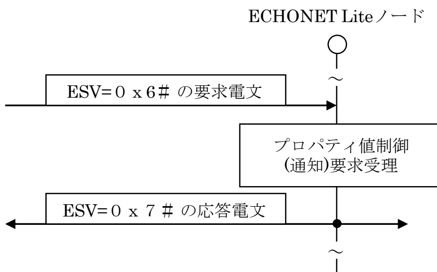
図 4-4 ESV=0x6a (a : 1～3, E) 要求受信時の基本シーケンス
