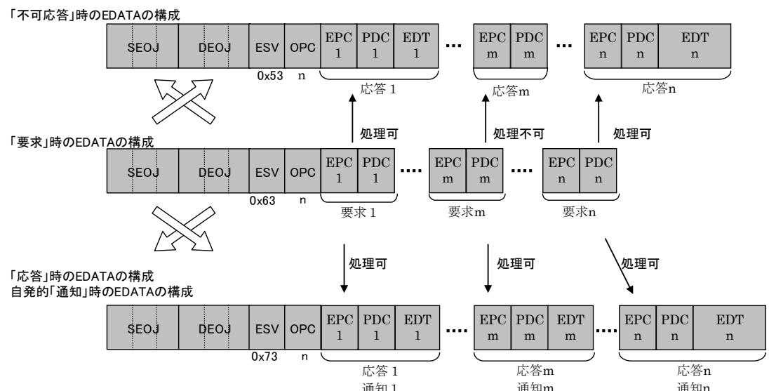
図 3-1 1 プロパティ値通知サービス時の EDATA の構成
