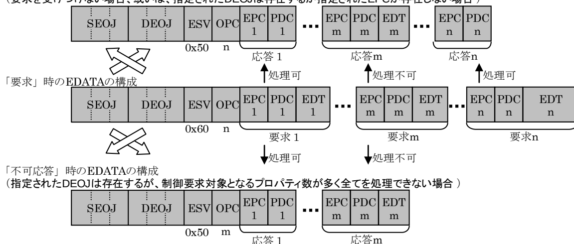
図 3-7 プロパティ値書き込みサービス（応答不要）時の EDATA の構成
