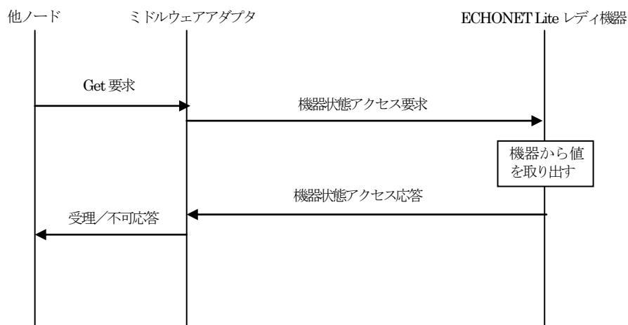
図 3-19 IAGetup の動作
