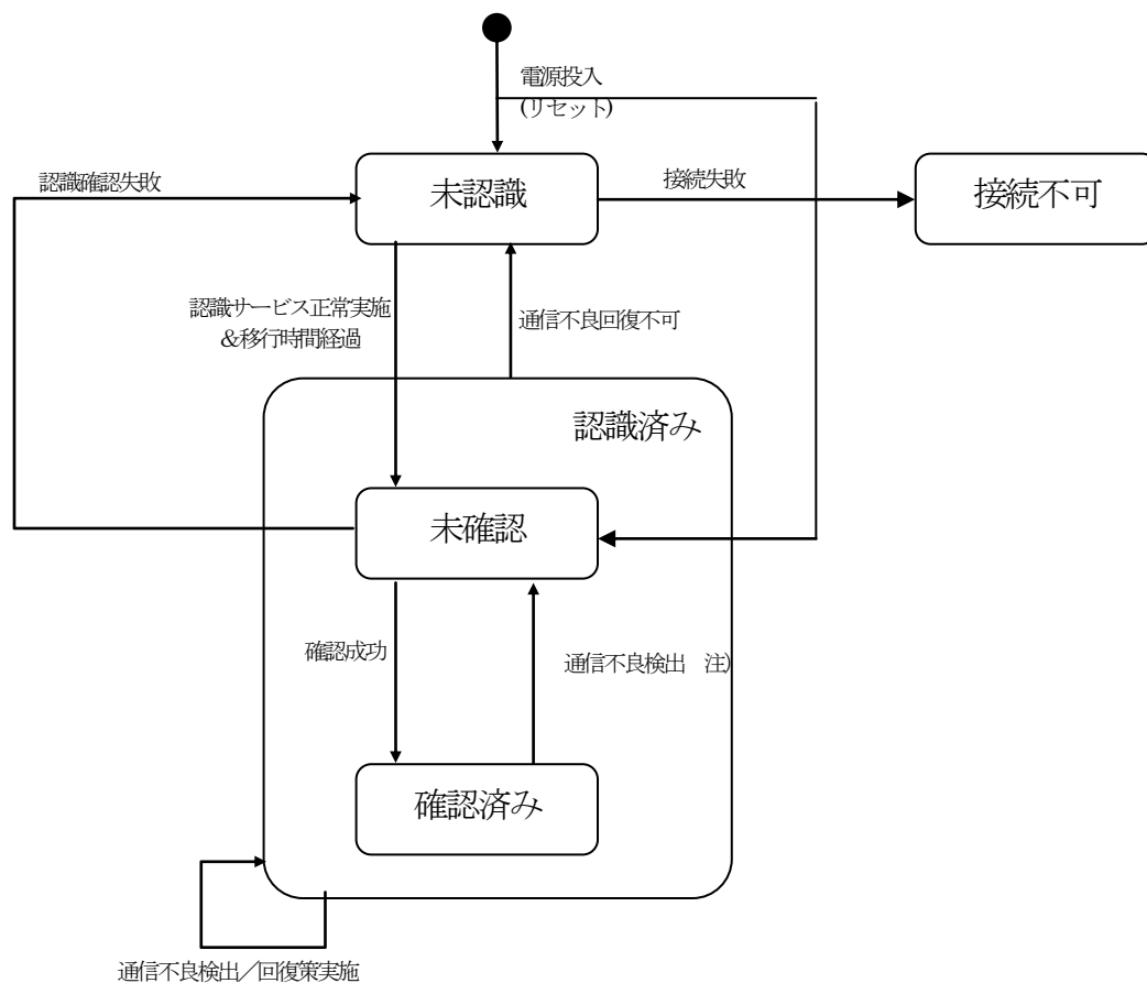
図 3-14 状態遷移
