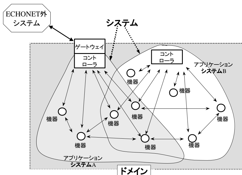
図 2-2 アプリケーションシステムの構成例と、ドメインの範囲
