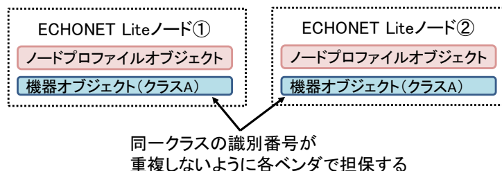
(2) 異なるノード上での同一クラスの機器オブジェクト搭載の例
